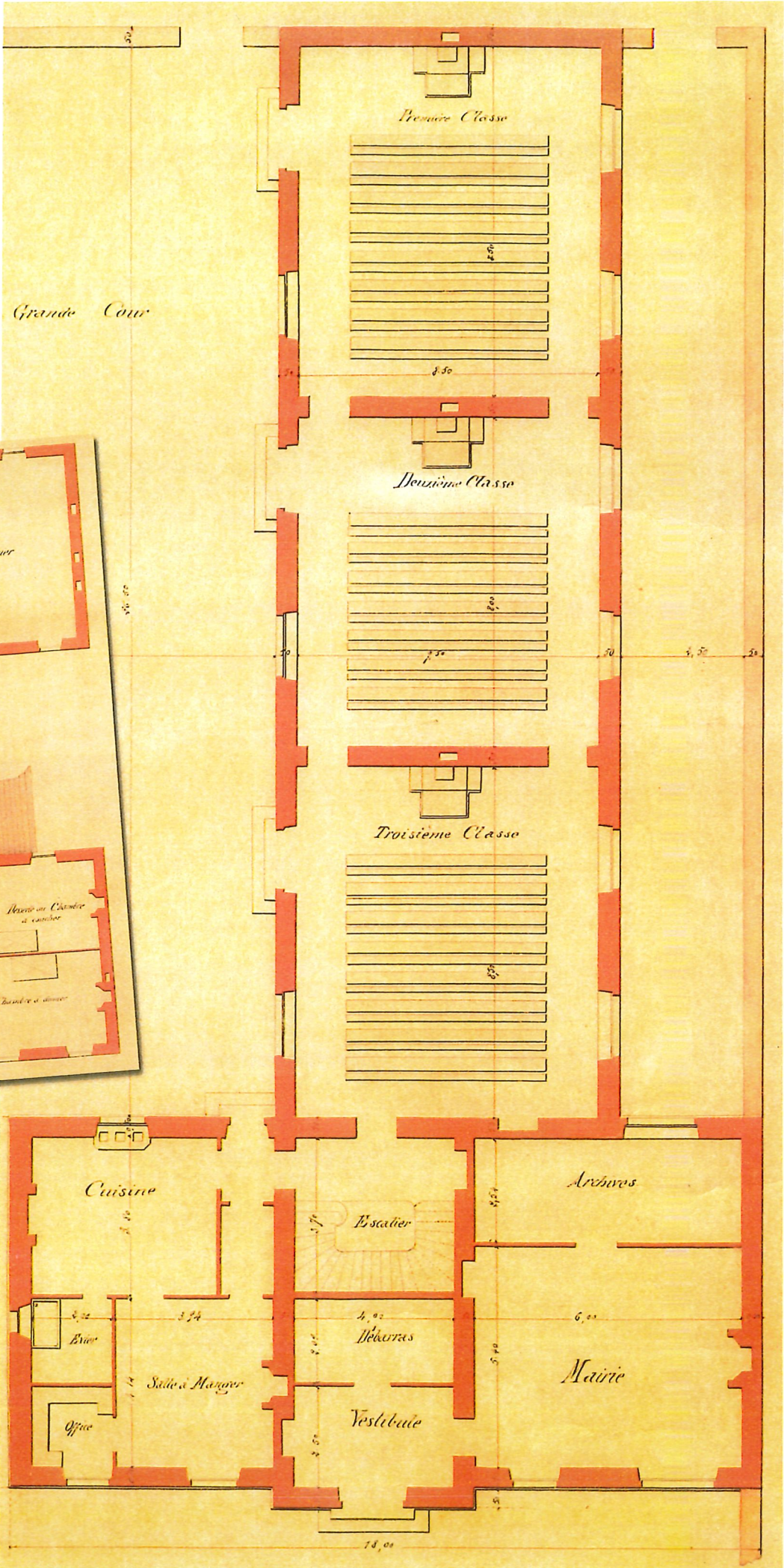
Plan du rez-de-chaussée
